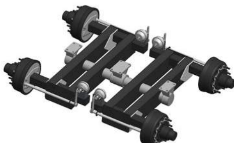
Балансировочная подвеска
